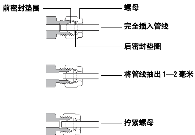
图 10 插入管线
