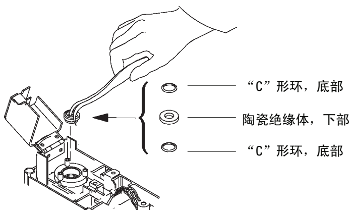
图7 NPD 下陶瓷绝热体和“C”形圈
