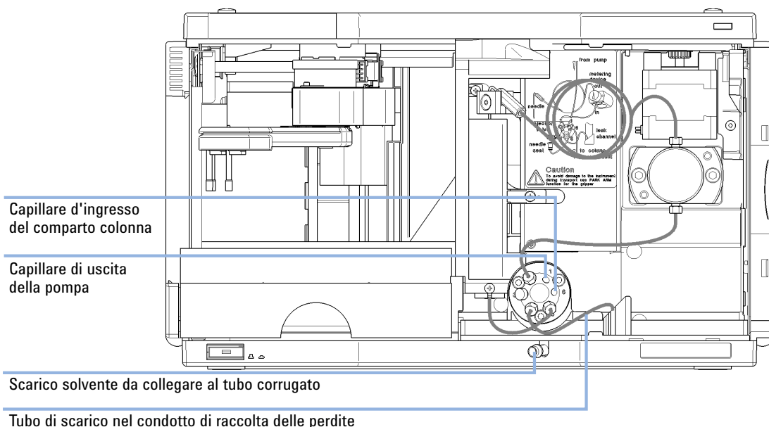
Figura 13 Collegamenti idraulici
