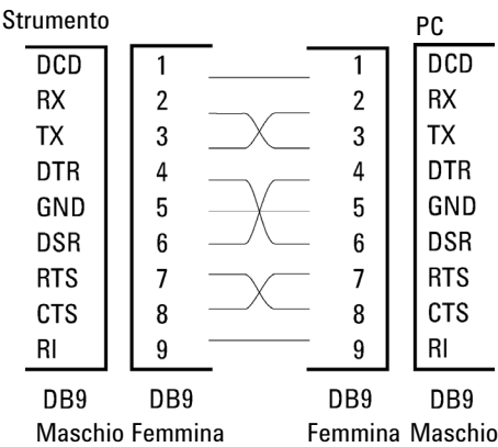
Figura 21 Cavo RS-232
