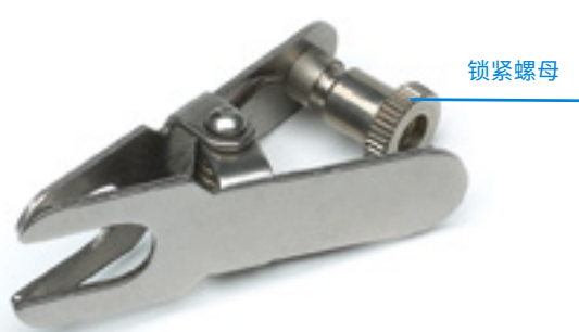
图 3a. 半可拆卸式和完全可拆卸式 ICP-OES 惰性炬管使用标准炬管固定夹
