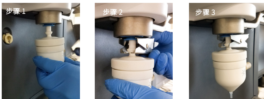
图 4. 将惰性雾化室安装到 MP-AES 惰性炬管上
